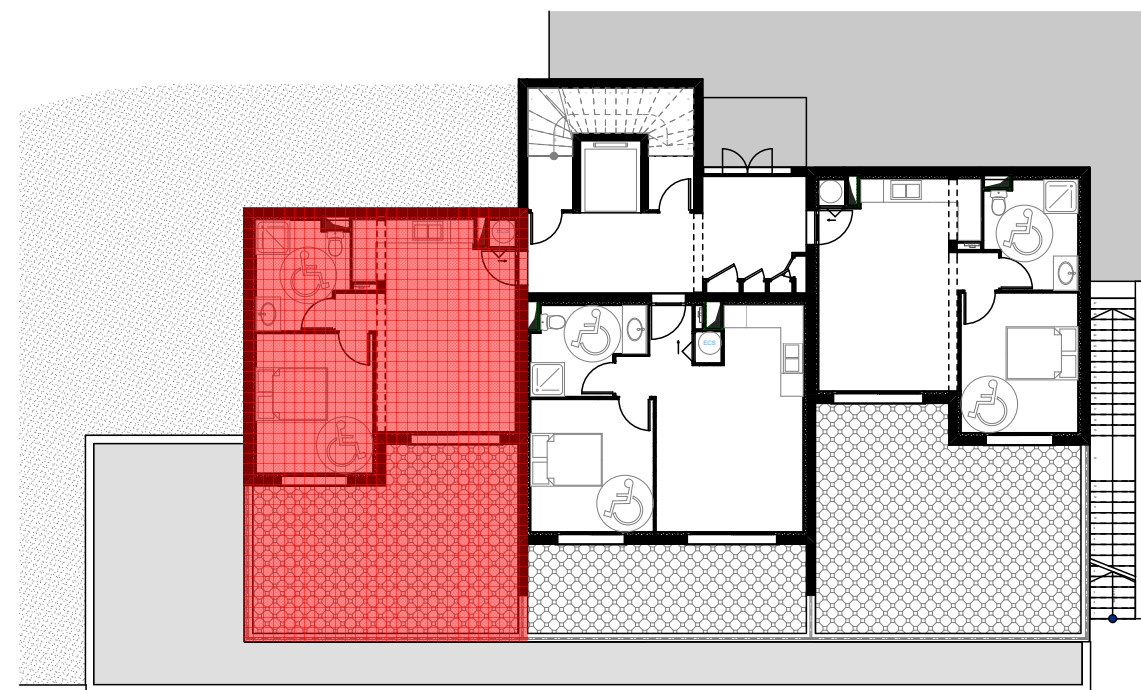
Plan d'étage courant R-1
